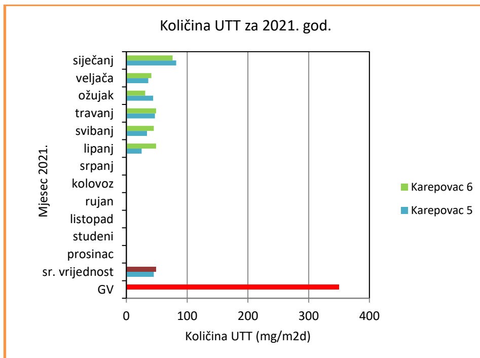
Slika 3. Količina UTT na mjernoj postaji Karepovac u 2021.god
